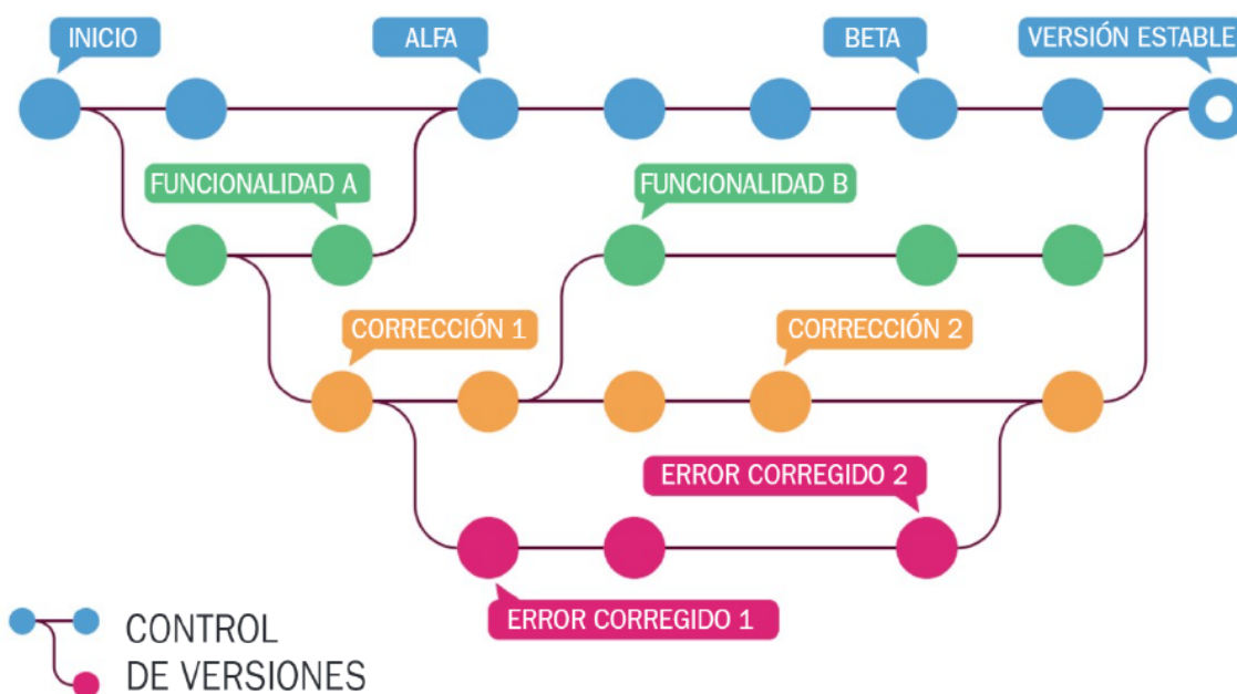
Figura 1.8. Ejemplo gráfico de las ramificaciones y fusiones de ramas en un proyecto con Git.
